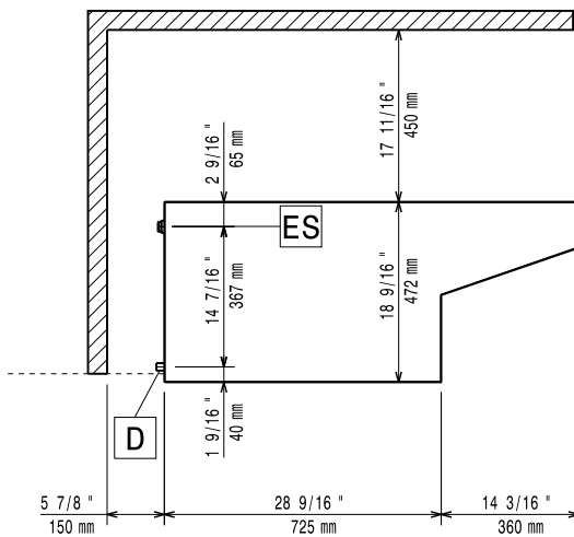
Boven aanzicht
